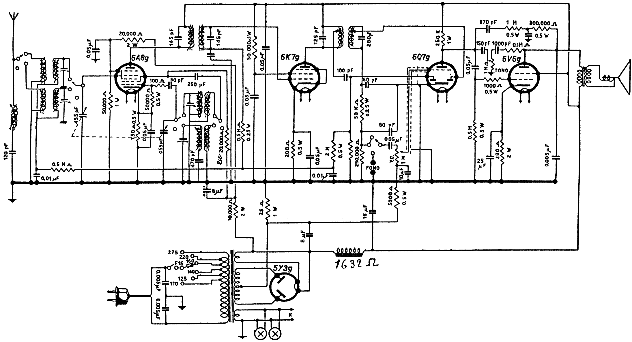
10 - COMPAGNIA GENERALE DI ELETTRICITÀ - MODELLI 255 e 355. Gamme di ricezione: da 190 a 580 m e da 17 a 50 m. Blocco alimentazione su telaio a parte. Potenza: 4,2 W. MF: 468 kc/s. Il mod 355 differisce dallo schema per avere in più una EM4, indicatrice di sintonia. V. Tabella tensioni in « Note di servizio ».
